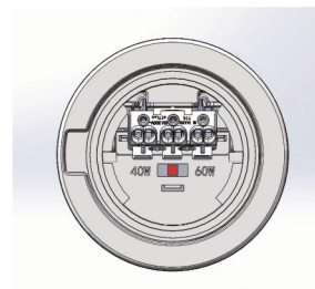
PRZEŁĄCZANIE MOCY W LAMPIE
